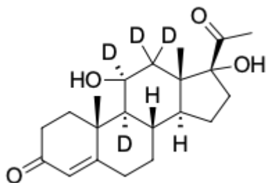
Структура 21-Дезоксикортизол-d4
