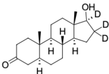
Структура 5α-дигидротестостерон-d3
