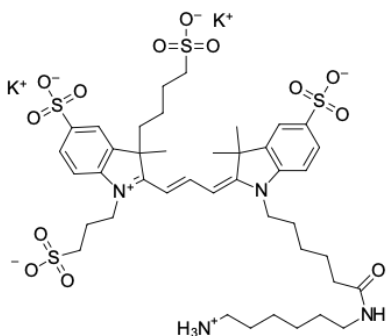
Структура AF 555 амина
