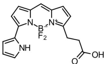
Структура BDP 576/589 карбоновой кислоты
