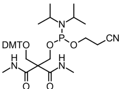
Структура амидита фосфата
