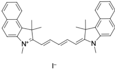
Структура Суанине5.5 диметила
