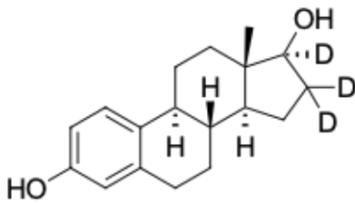
Структура Эстрадиол-d3
